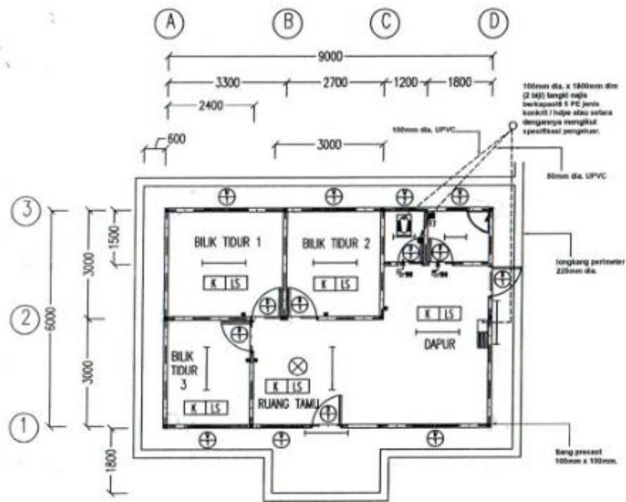
PELAN LANTAI
